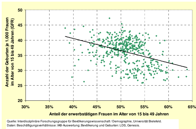
Schaubild 1: Streudiagramm des Anteils der erwerbstätigen Frauen (31.12.2002) und der allgemeinen Fertilitätsrate ( \bar{\sigma} 2001-2003) für alle 439 Land- und Stadtkreise in Deutschland
